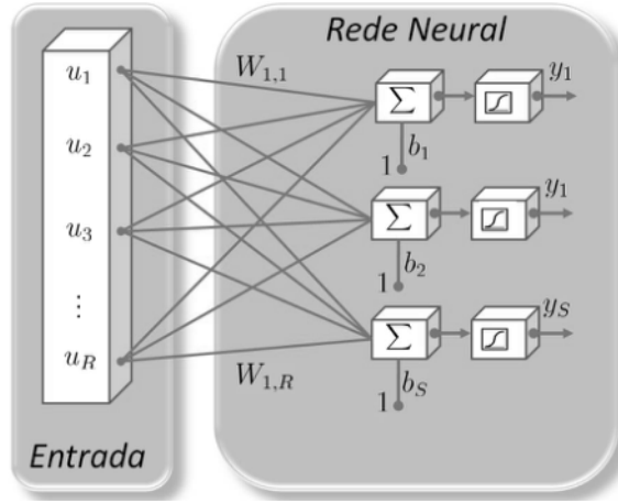
Figura 13 – Rede Neural Artificial com uma camada
