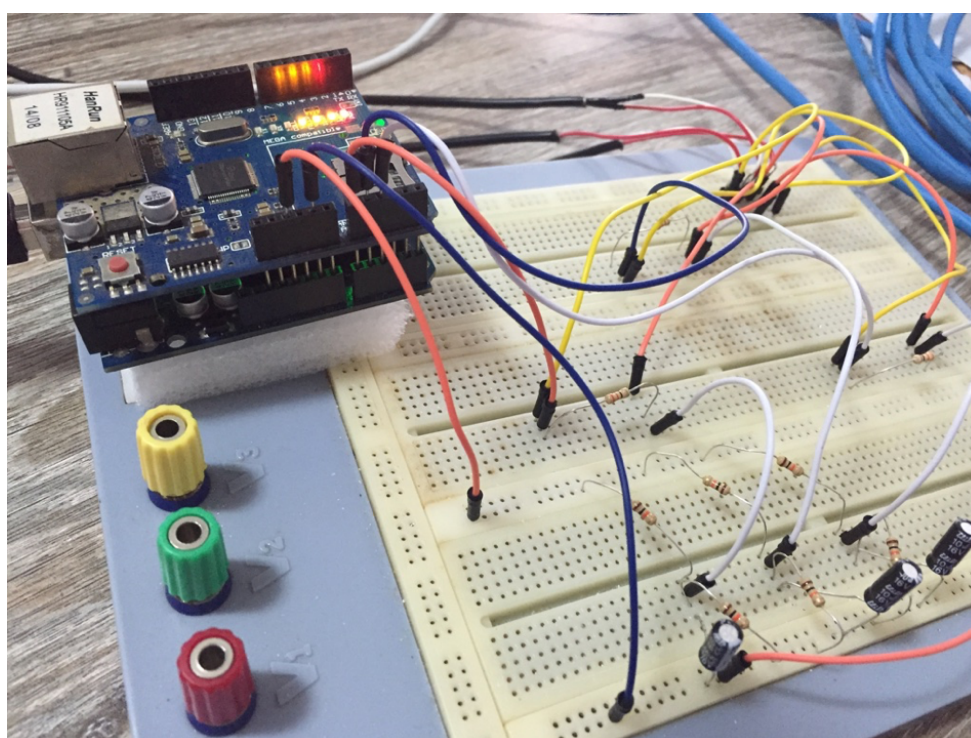
Figura 24 – Testes com circuito de recepção do sinal de corrente
