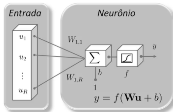
Figura 11 – Modelo de um neurônio
