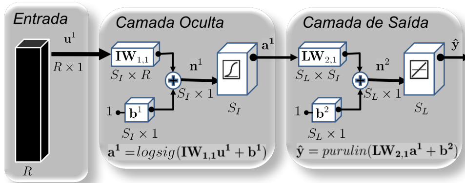
Figura 14 – Estrutura para uma Rede Neural Feedforward
