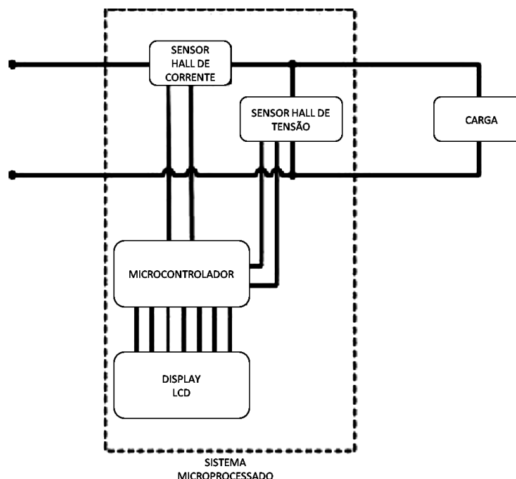
Figura 5 – Funcionamento básico de um medidor eletrônico
