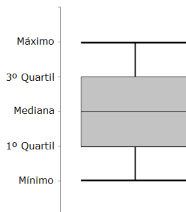
Figura 8 – Exemplo de um Gráfico de Caixa
