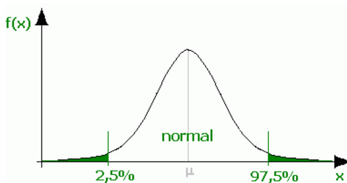
Figura 9 – Exemplo de uma distribuição normal
