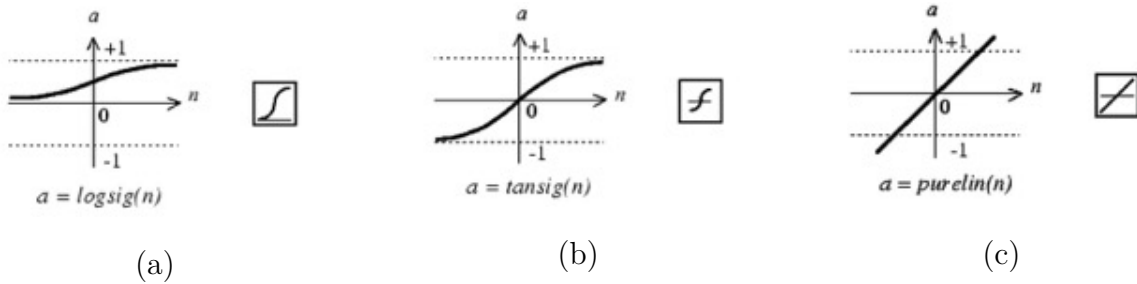
Figura 12 – Funções de transferências para Redes Neurais multicamadas
