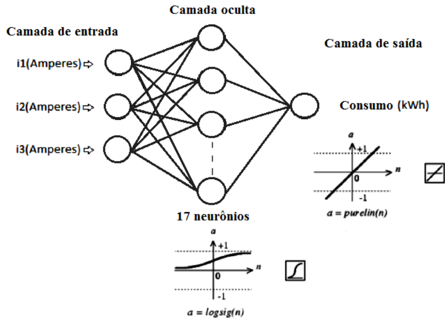
Figura 21 – Arquitetura da RNA feedforward desenvolvida
