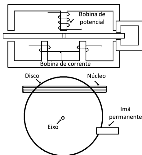
Figura 3 – Mecanismos do medidor eletromecânico de energia elétrica
