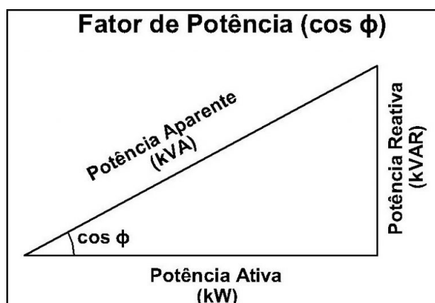
Figura 16 – Relação entre as três componentes da potência elétrica e o fator de potência
