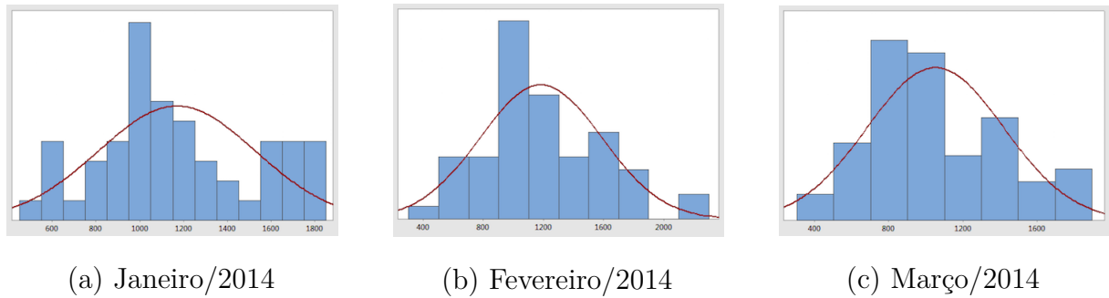
Figura 19 – Distribuição Normal para os dados sem outliers
